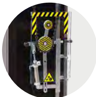
Air pressured adjustable chain tensioner Régulateur de tension de chaîne réglable à air comprimé Tensor de cadena ajustable neumáticamente
